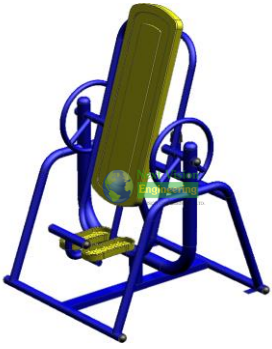
FT-58 อุปกรณ์บริหารแขน-หน้าท้อง (แบบยืน) กว้าง 100 ซม. ยาว 100 ซม. สูง 160 ซม.
