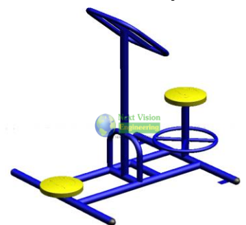
FT-57 อุปกรณ์บริหารเอว-สะโพก (แบบนั่ง-ยื่นบิดเอว) กว้าง 100 ซม. ยาว 100 ซม. สูง 120 ซม.
