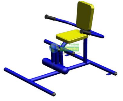
FT-33 อุปกรณ์แก้ปวดเข่า (แบบสลักขา) กว้าง 1.00 เมตร ยาว 1.00 เมตร สูง 0.80 เมตร
