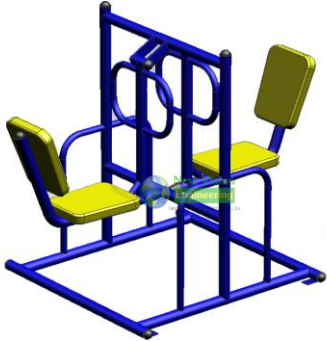
FT-61 อุปกรณ์บริหารขา-เข่า-น่อง (แบบขาดันยกตัว) กว้าง 160 ซม. ยาว 150 ซม. สูง 100 ซม.
