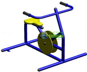
FT-04 อุปกรณ์บริหารข้อเข่า-ขา (แบบจักรยานล้อเหล็กนั่งตรง) กว้าง 1.00 เมตร ยาว 1.00 เมตร สูง 0.90 เมตร
